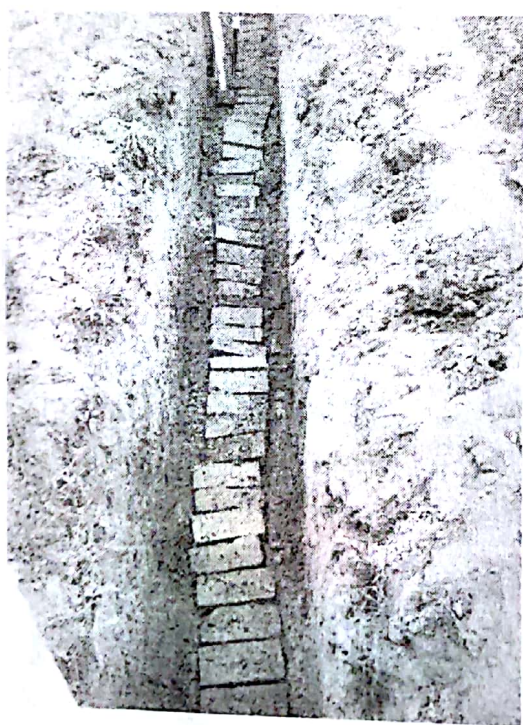
42 区直流电缆沟回填
