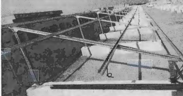
瑞金市“十二五”贫困村光伏扶贫扩面工程 厂房屋顶直流电缆敷设20180813
