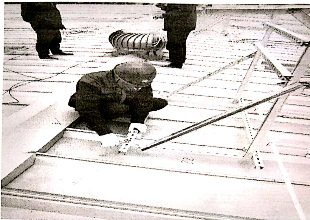
10号屋面汇流箱支架安装
