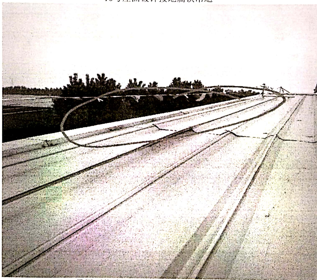
10号屋顶临边安全防护不规范 (01)
