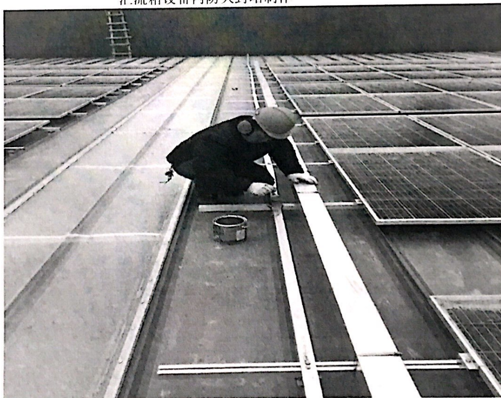
D号屋面镀锌扁铁防腐处理
