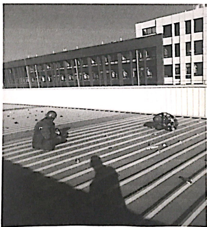
屋面光伏区夹具安装（1）
