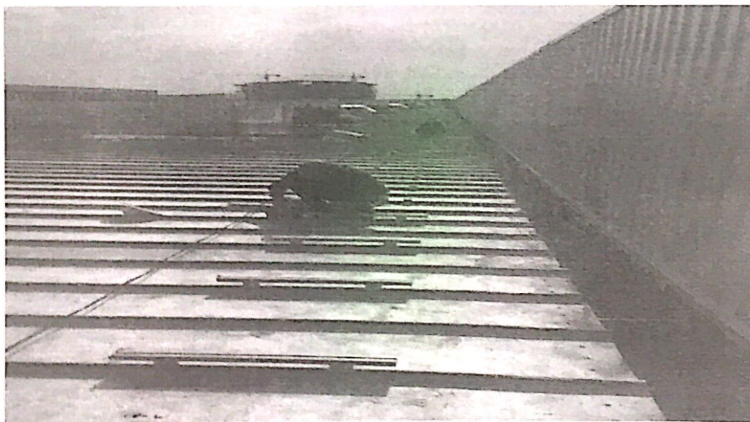
2#屋面格栅通道支架、檩条安装
