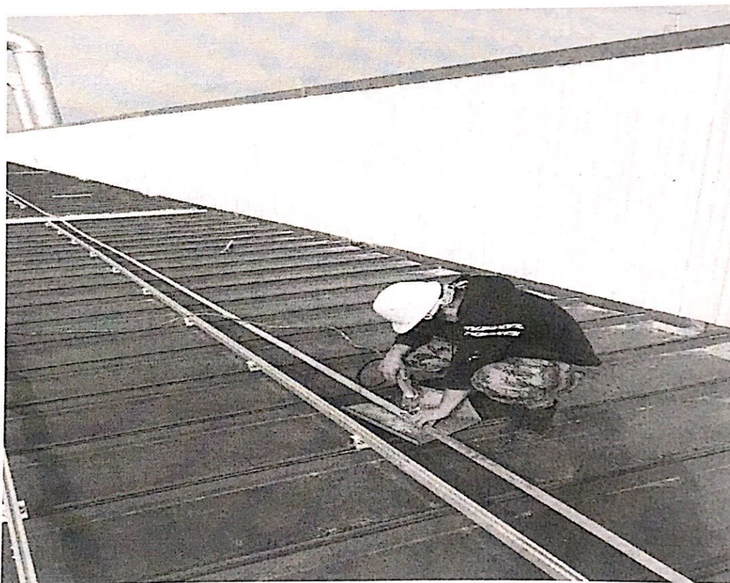
1#屋面光伏区镀锌接地扁铁焊接
