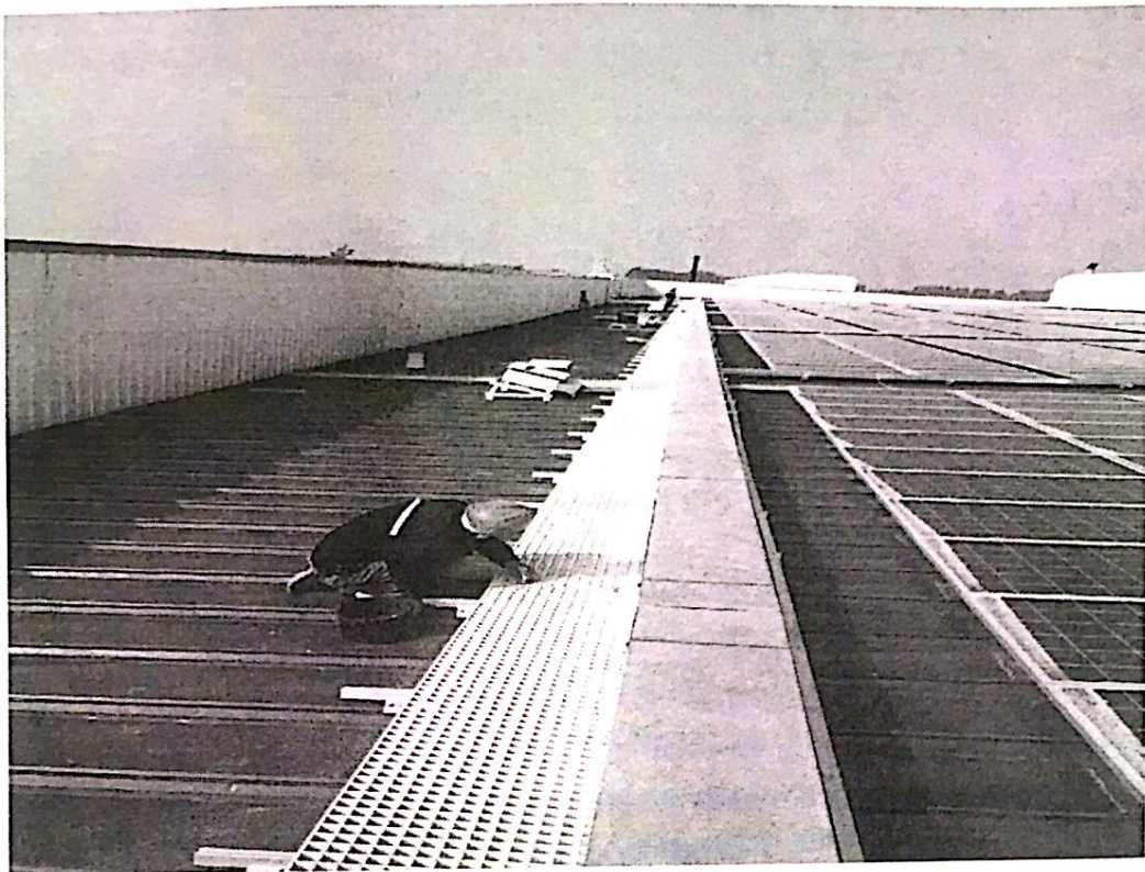
1#屋面光伏区格栅检修通道安装
