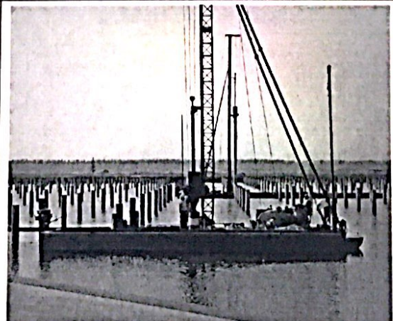
D 区打桩
