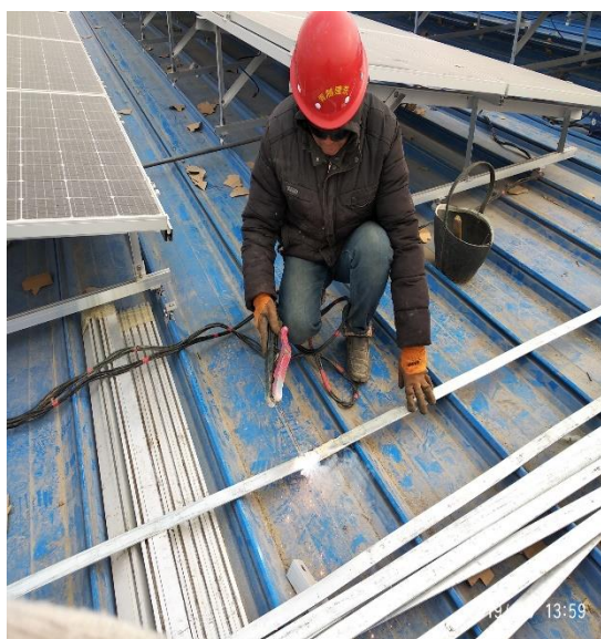
接地扁钢焊接
