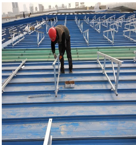
安装支架
