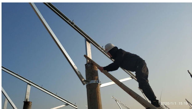
立柱焊接检查
