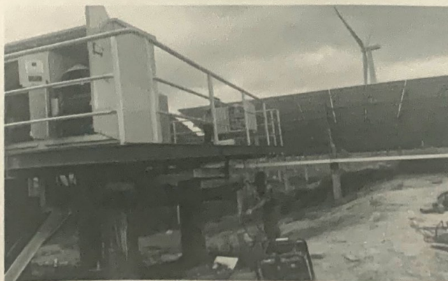
39#通讯电缆接线
