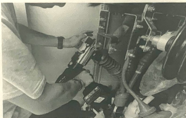
集电线路进入 39#箱变高压电缆头制作
