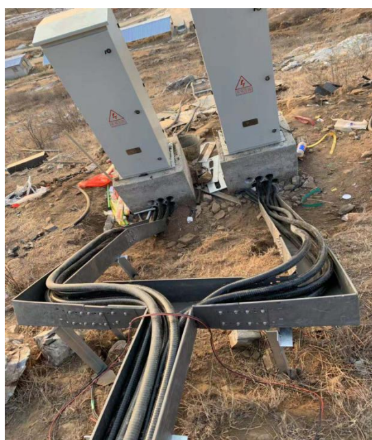
桥架安装
