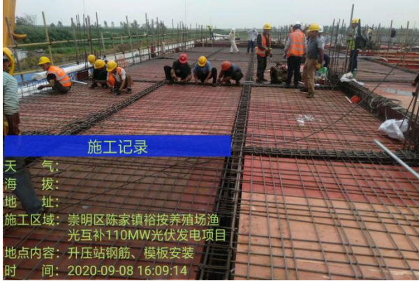
升压站二层底板 钢筋绑扎
