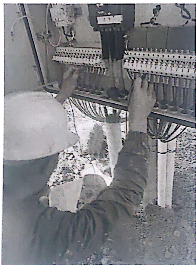
汇流箱接线电压测试
