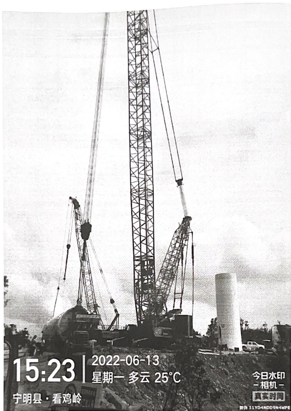
17#风机吊装
