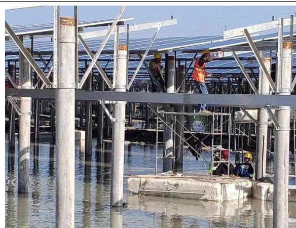
一标段光伏区支架、组件安装
