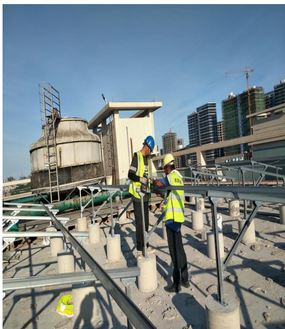
支架安装
