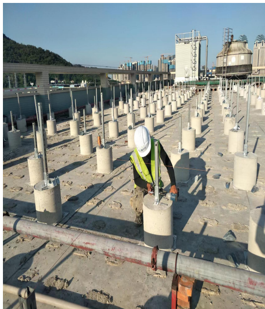
支架安装
