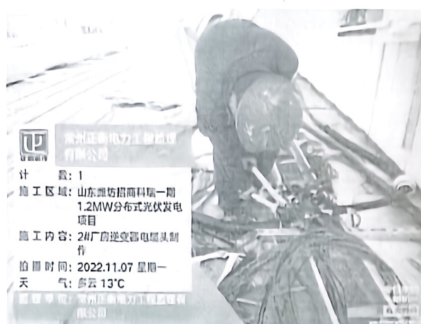
2#厂房逆变器电缆头制作
