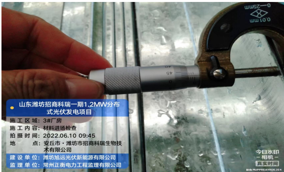
檩条检查
