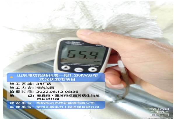
镀锌层测量
