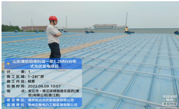
支架检查
