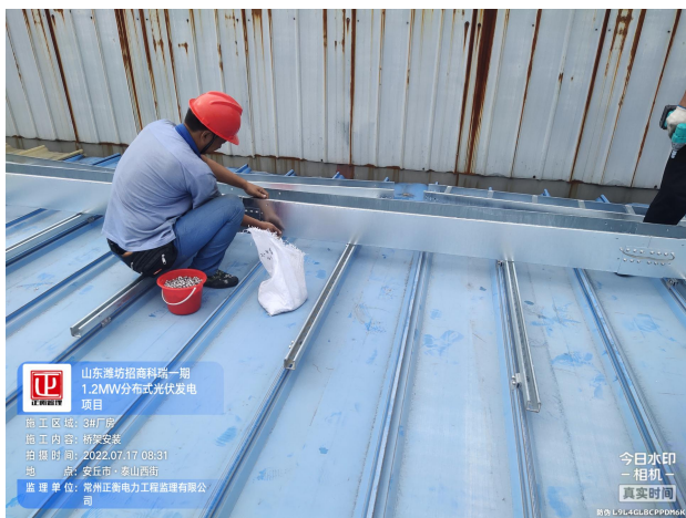
电缆桥架对接
