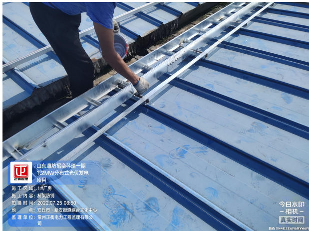
桥架防腐
