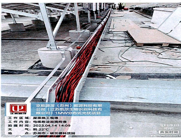
电缆敷设
