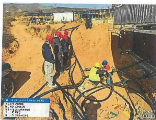
洪池地块 29 箱变侧交流电缆头制作
