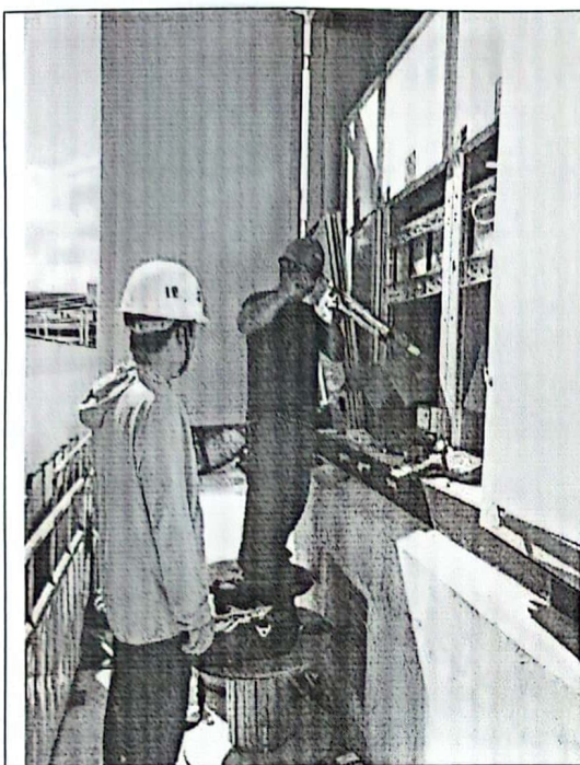
箱变高压电缆终端头制作
