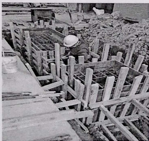
承台基础支模
