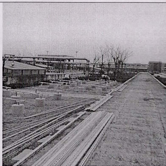
水池钢结构中部植筋
