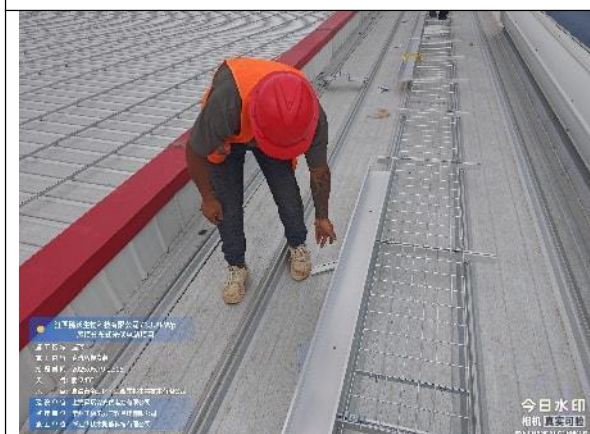
直流桥架安装
