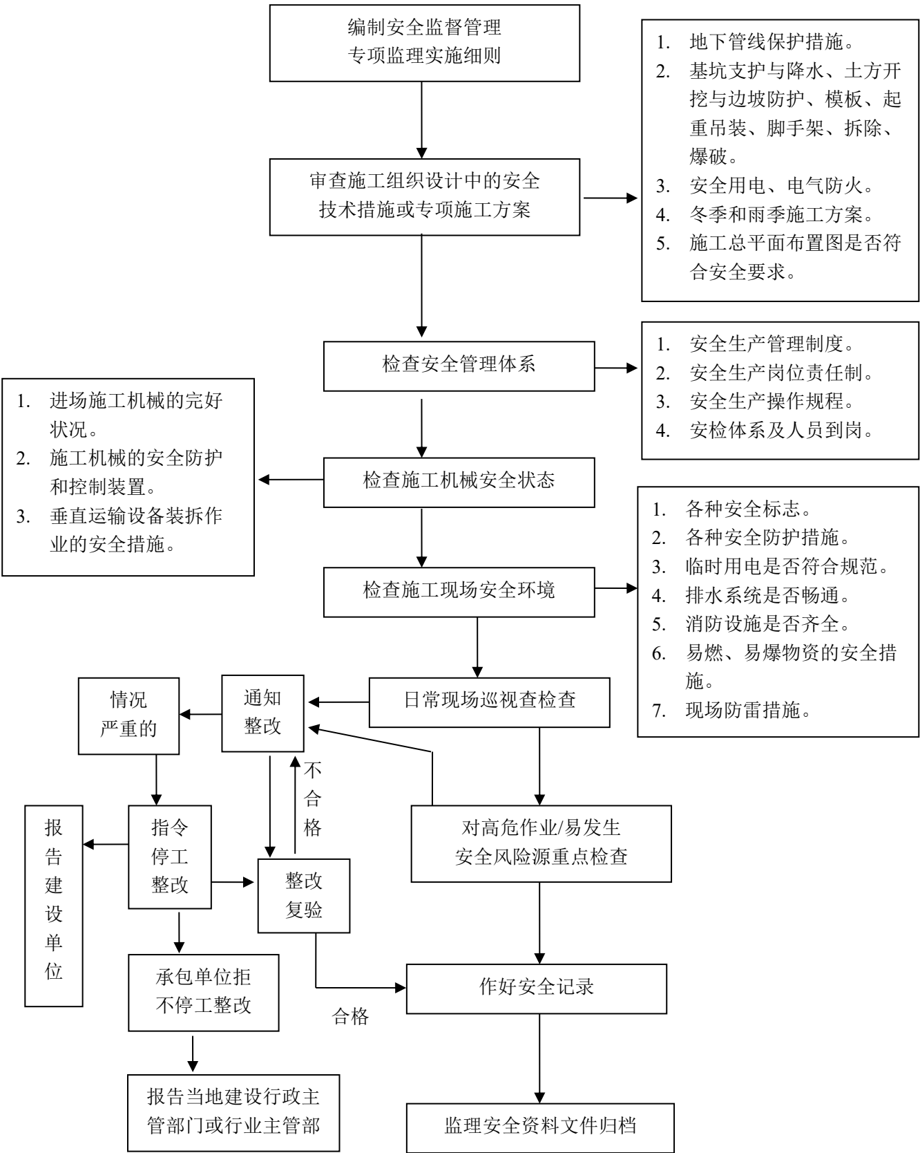
施工阶段工程安全监督管理程序框图
