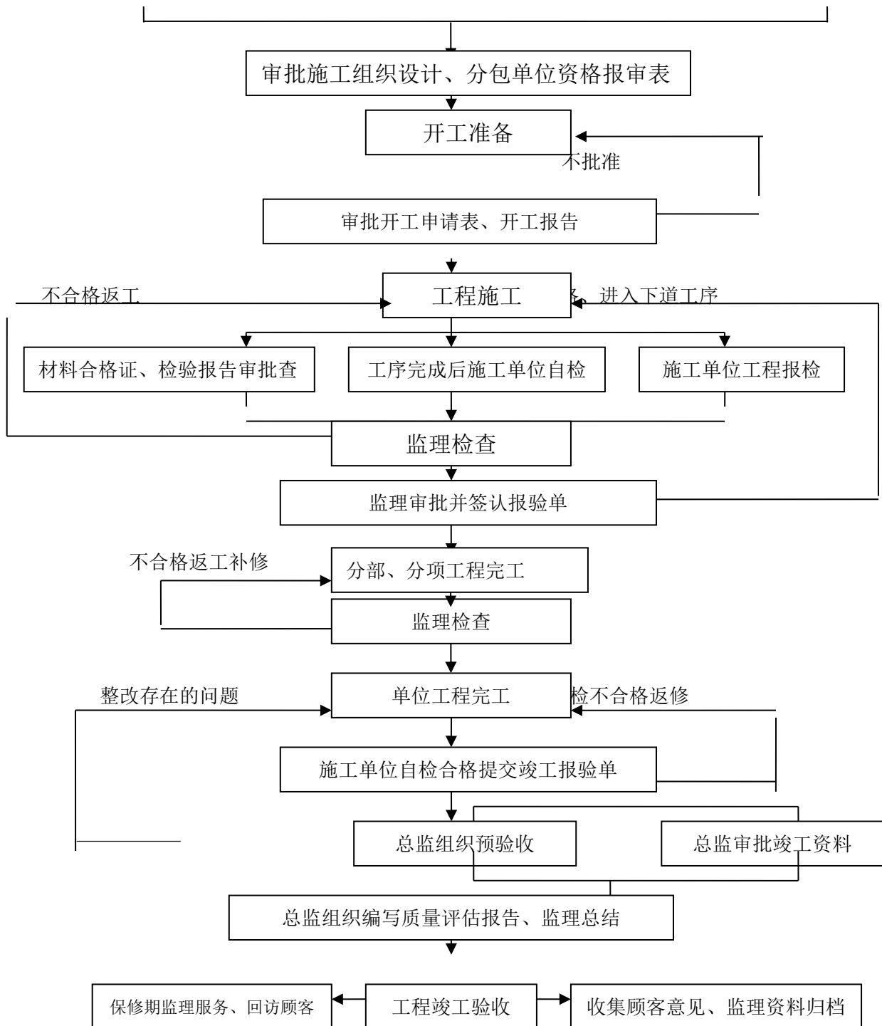
(监理工作流程图之二)
