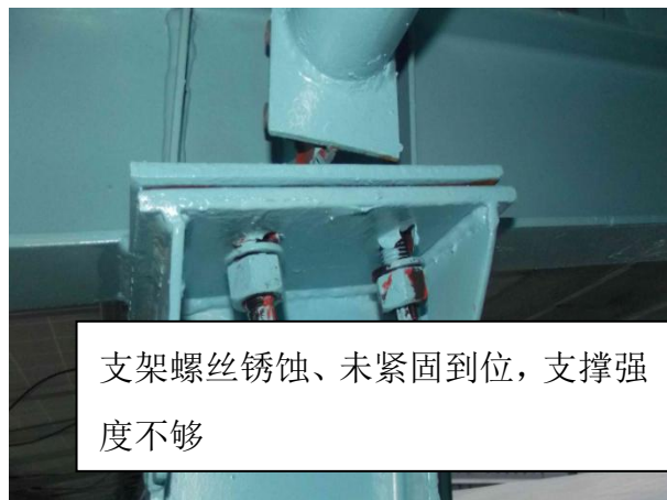
支架接头安装不符合要求，抗风等级不够
