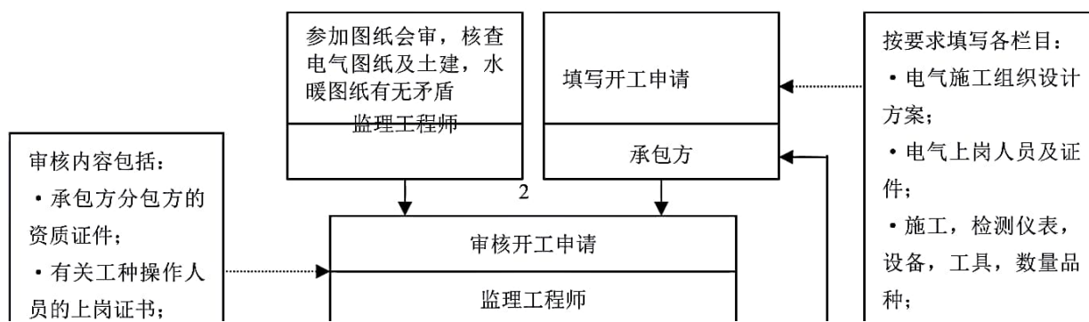
电气安装工程质量监理的工作流程
