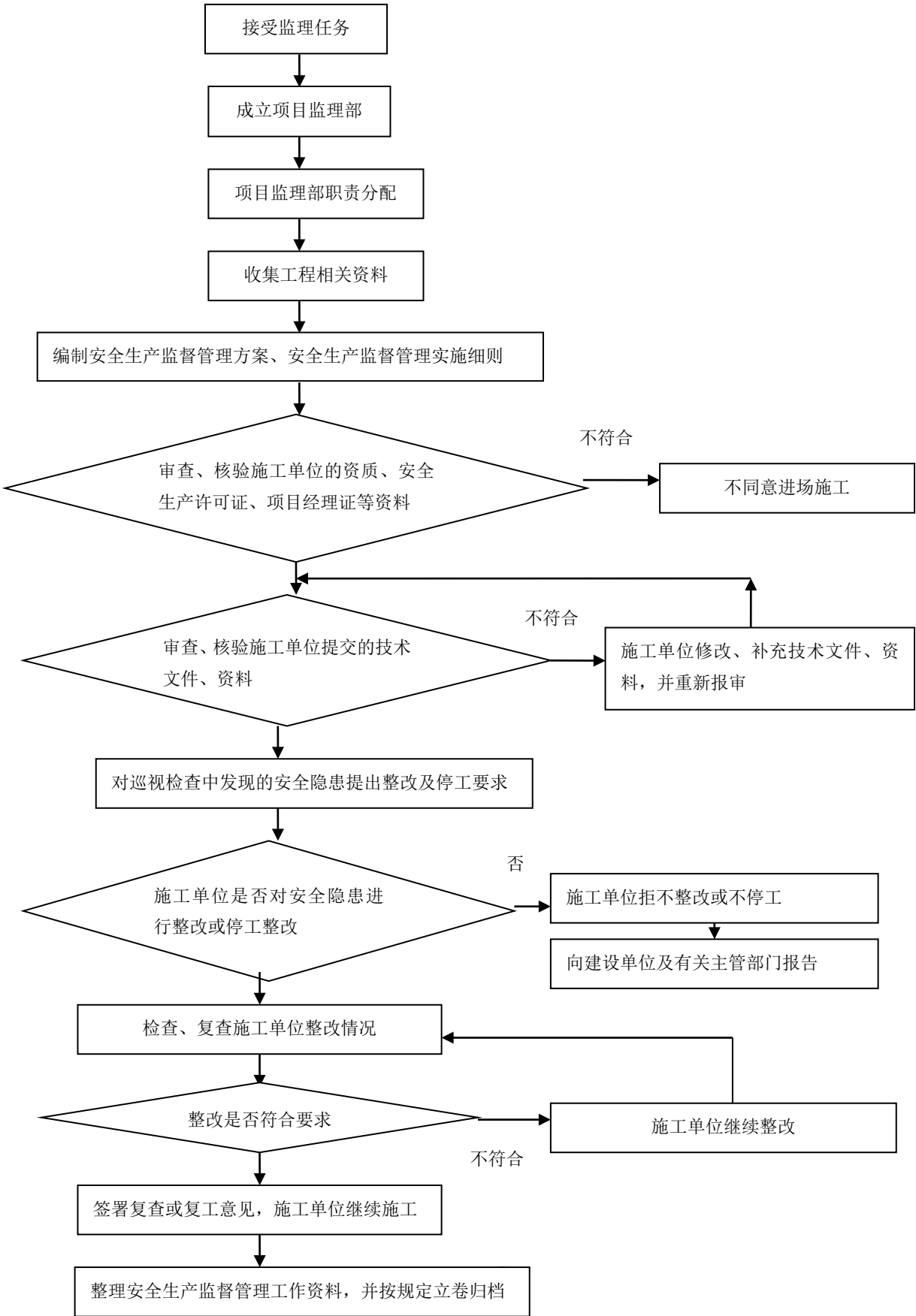
图 B.1 建 设 工 程 安 全 监 督 管 理 工 作 程 序 框 图
