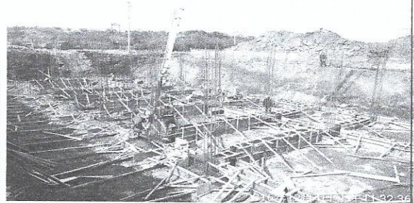
配电装置楼基础框架梁浇筑
