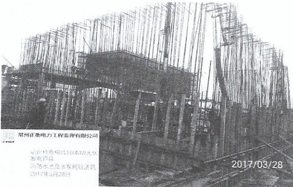
水泵房及消防水池地梁、构造柱砼浇筑
