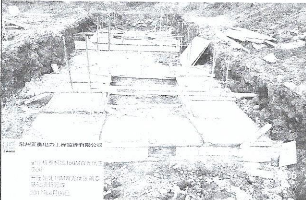
光伏区箱变基础承台浇筑
