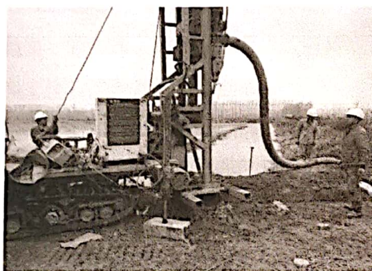
钻机就位
