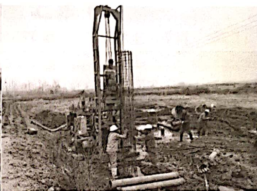
下钢筋笼
