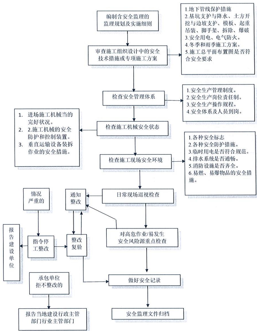
图 B.3 施工阶段工程安全监理程
