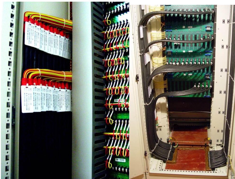
图五 盘内电缆绑扎样板图
