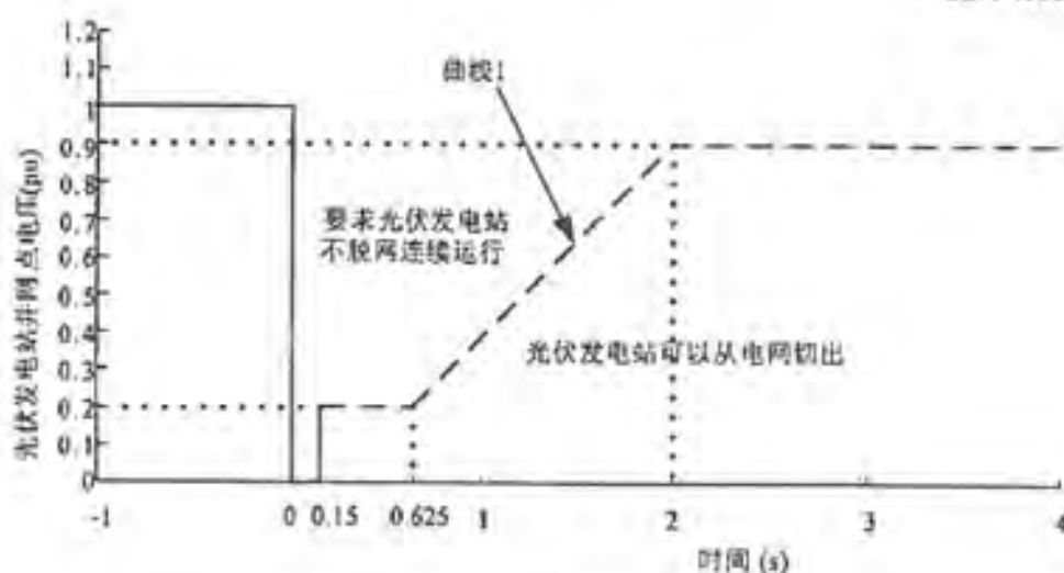
图1 光伏电站的低电压穿越能力要求
