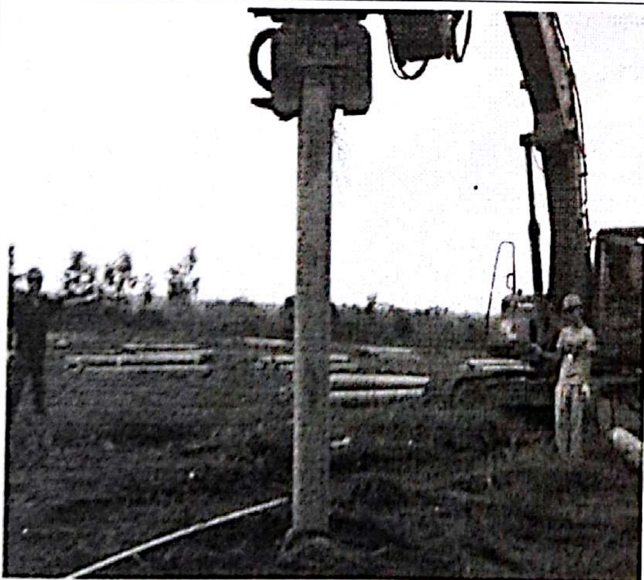
管桩施工
