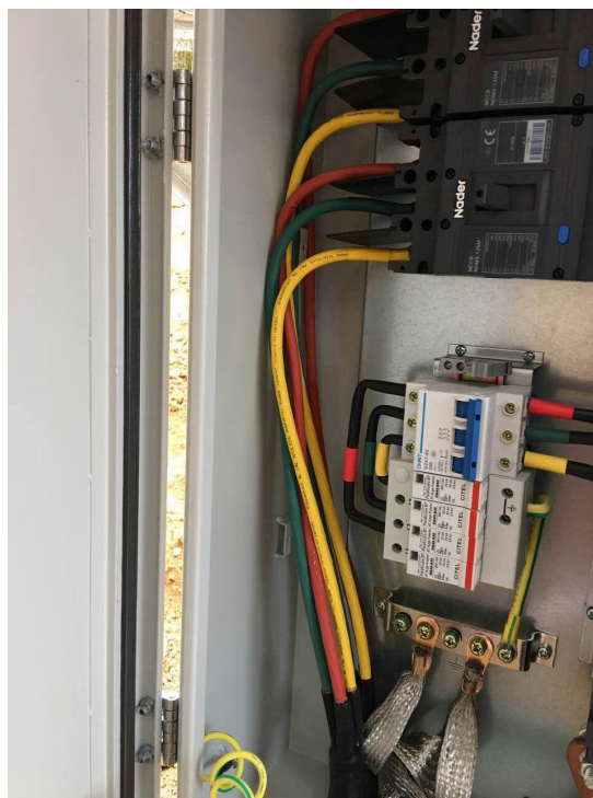
2017 年 11 月 22 日红联光伏区 12 子阵逆变器接线
