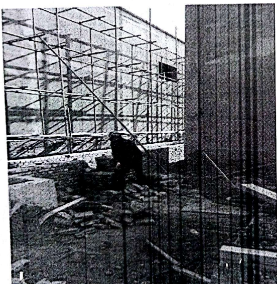
电气楼外砖砌电缆沟
