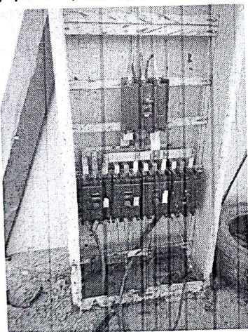
P2 区三级配电箱无保护措施，且接线杂乱
