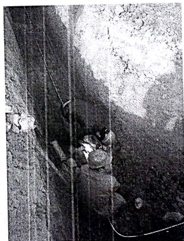
焊接 80x8 接地扁铁
