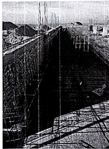
P3 区升压站 SVG 基础钢筋绑扎
