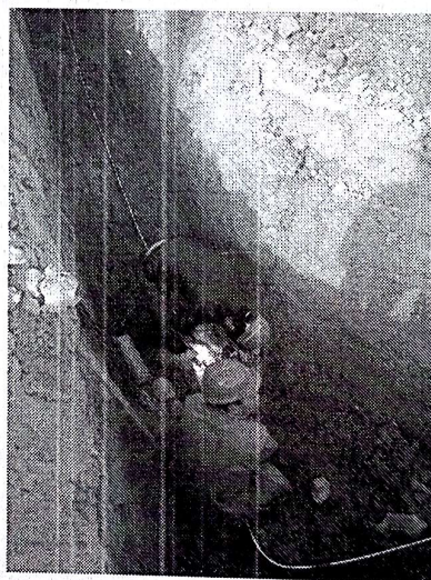
焊接 80x8 接地扁铁
