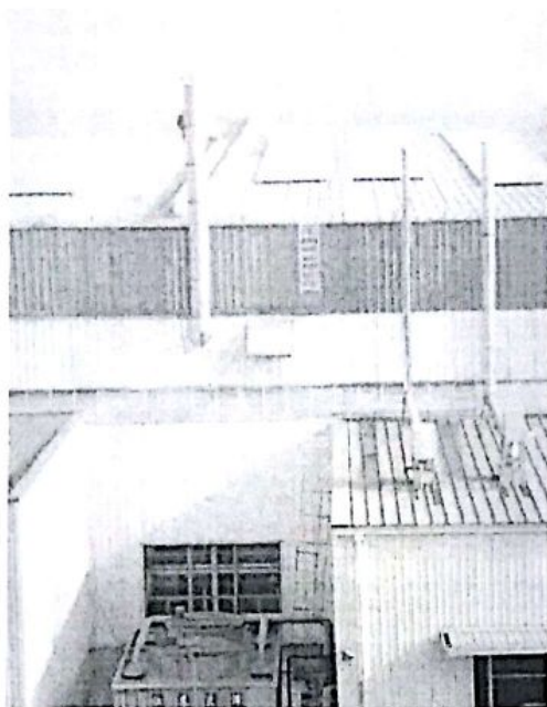
一期垂直桥架安装
