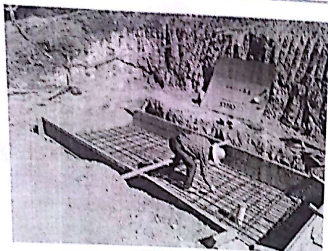
箱变基础施工
