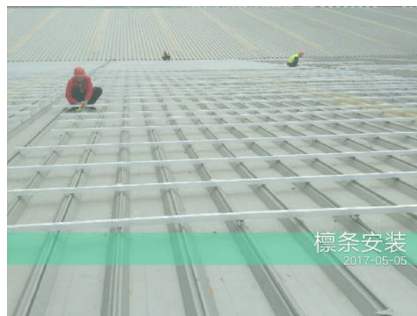
檩条安装
