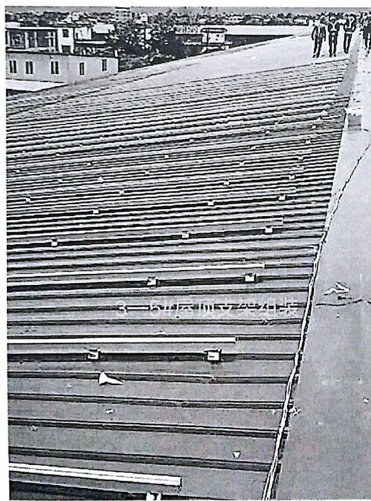
3—5#屋顶支架组装
