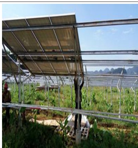
20 区光伏板安装
