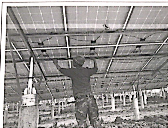
23 区 1×4 平方线展放
