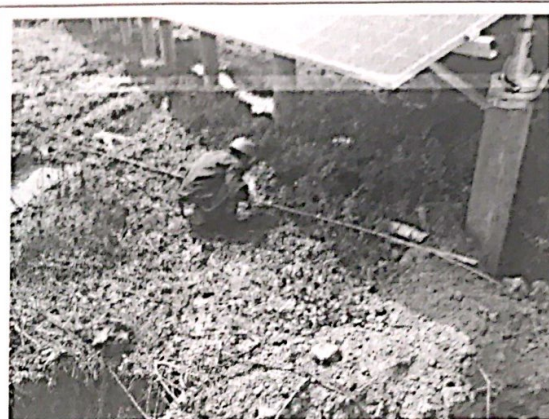
28 区接地扁铁焊接
