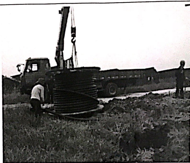
32 区高压电缆敷设
